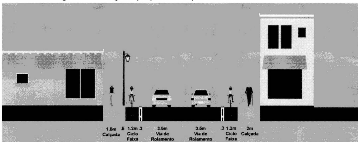
Figura 42 - Seção tipo pista de aproximadamente 10 metros
