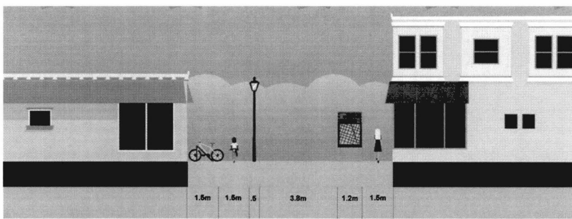
Figura 25 – Seção transversal esquemática para vias compartilhadas comerciais com caixa de 10 metros
