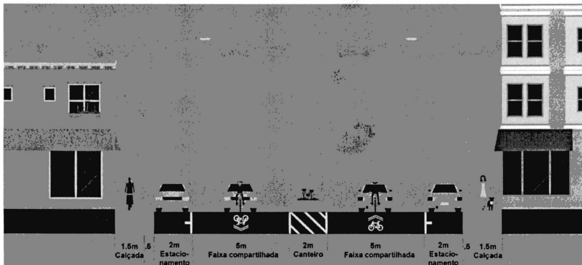
Figura 43 - Seção tipo pista de aproximadamente 14 metros
